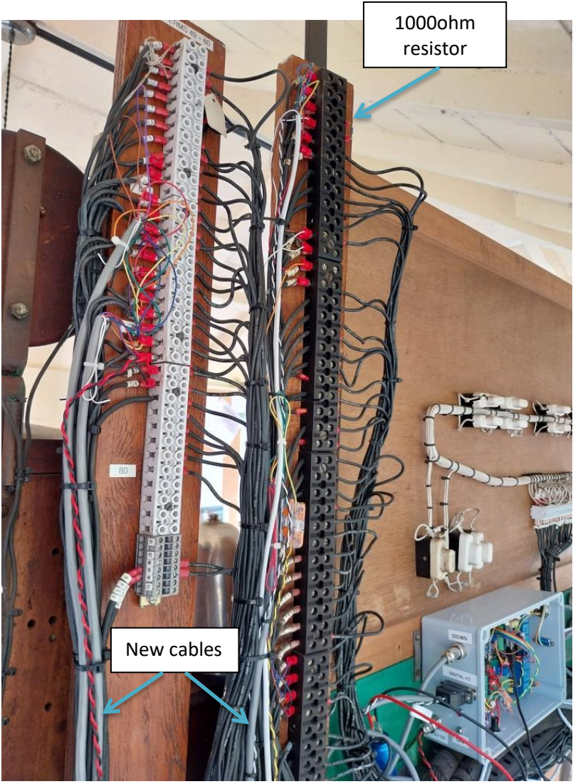
New Wiring
